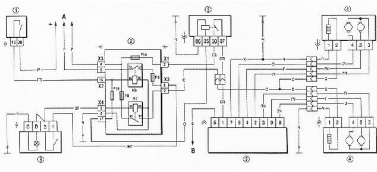
Схема включения элетроуправляемых зеркал
